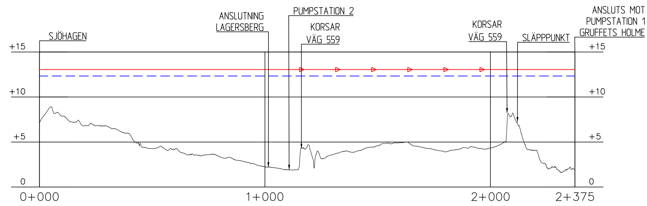
PROFIL: Alt 1 Ledningslinje Sjöheden-Gruffetsholme H-SKALA 1:10000 V-SKALA 1:250
