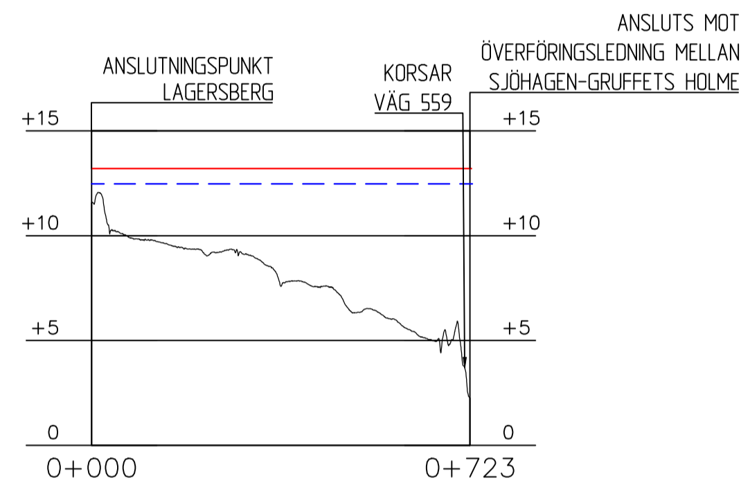
PROFIL: Alt 1 Ledningslinje Lagerberg-Sjöheden H-SKALA 1:10000 V-SKALA 1:250
