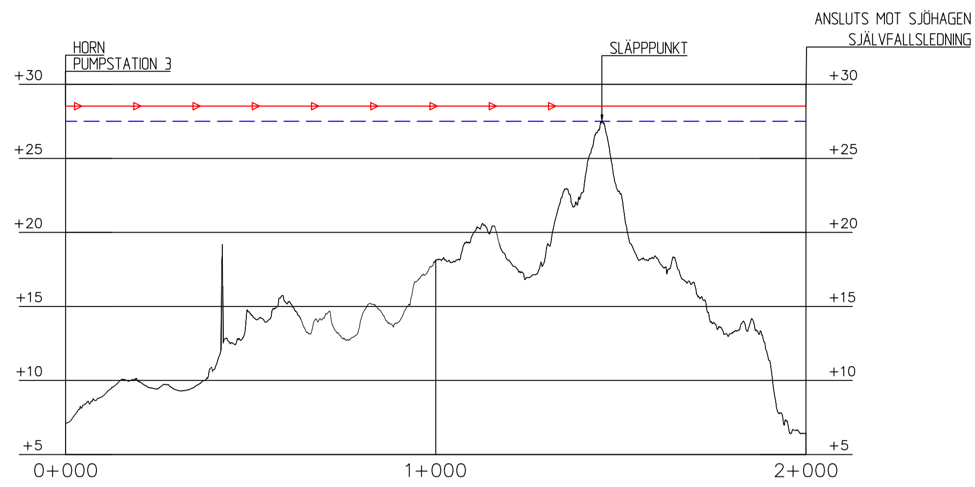
PROFIL: Alt 1 Ledningslinje Horn-Sjöheden H-SKALA 1:10000 V-SKALA 1:250
